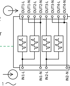
DGTM402 4 x 2 A TE dimmer module
